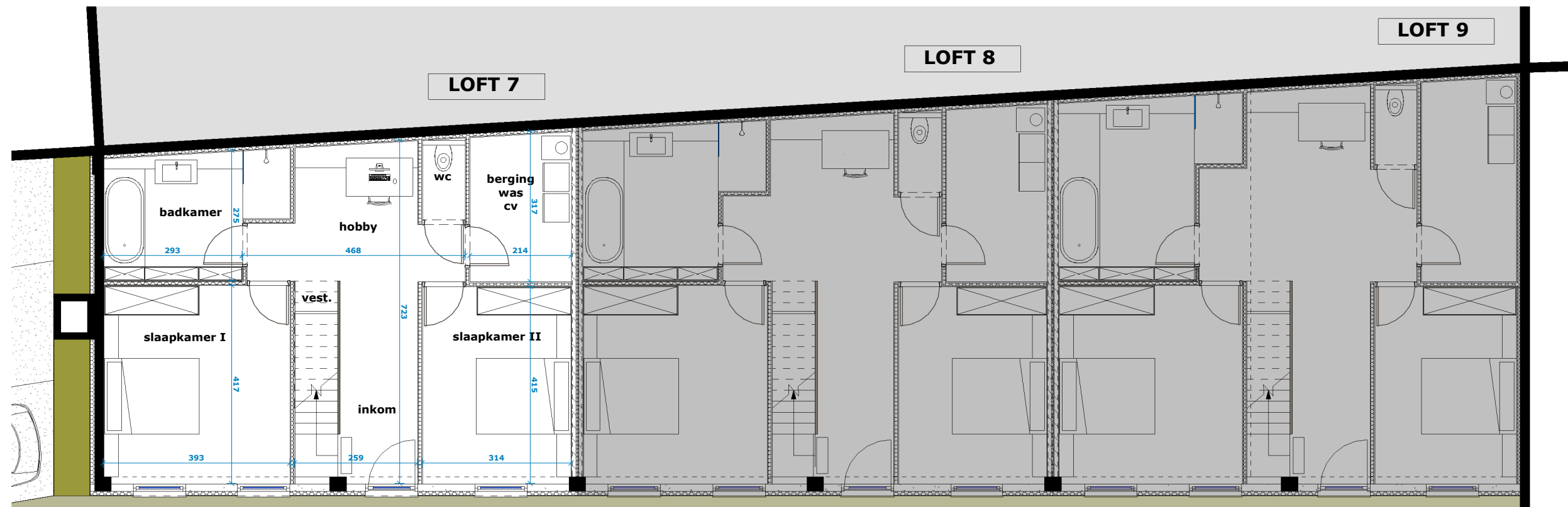
Gelijkvloers
